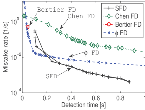
Fig. 9. WAN1: MR vs T_D
